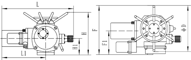
Рис.2 Вид приводов М-45-120
