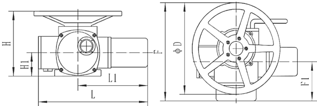
Рис.1 Вид приводов М-5-30
